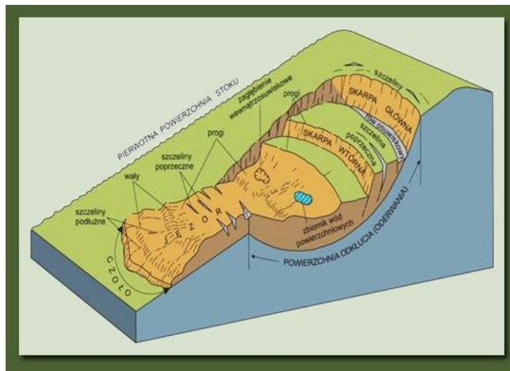
Rys. 1. Model osuwiska wraz z podaniem głównych elementów rzeźby osuwiskowej. („Instrukcja ...”, PIG, Warszawa, Grabowski i in., 2008), https://archiwum.mos.gov.pl/ .
